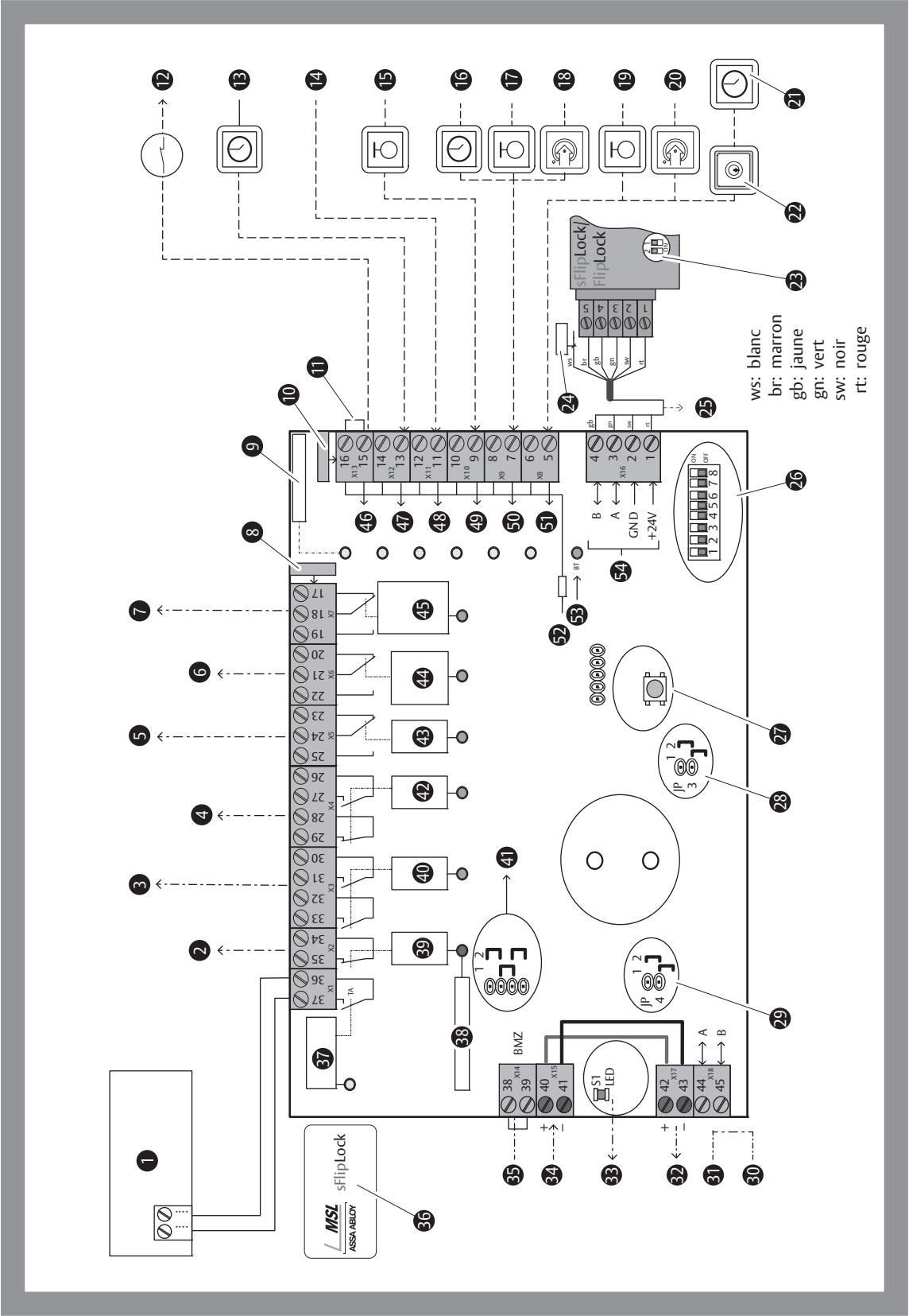
Fig. 11 : Schéma de raccordement mFlipLock e-access
