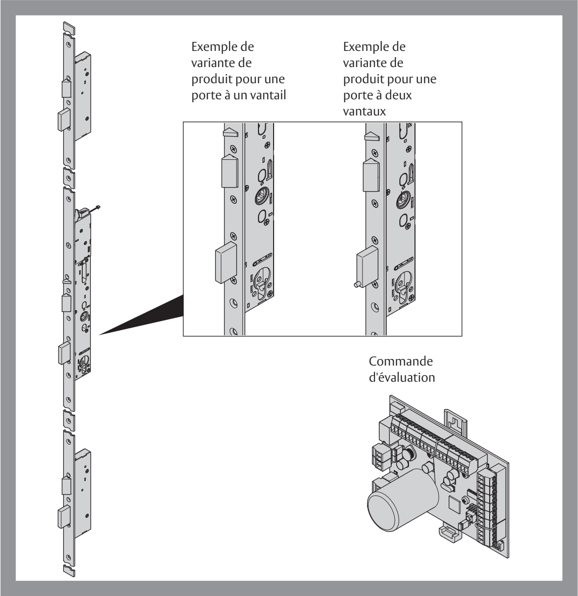
Fig. 1 : Serrure multipoints de sécurité antipanique mFlipLock access/e-access
