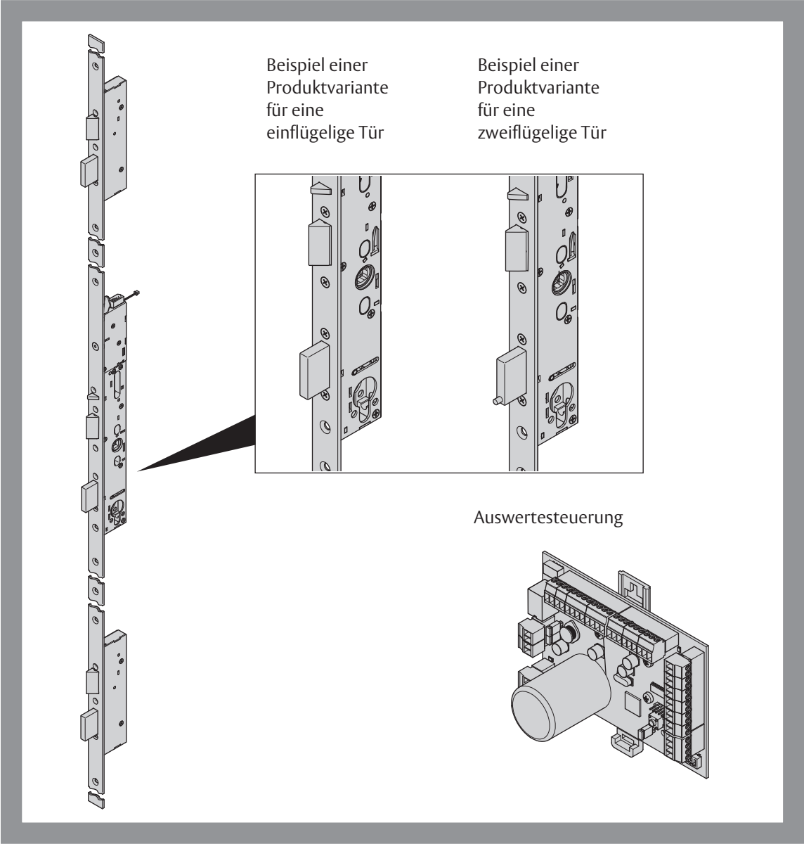
Abb. 1: Panik-Sicherheits- Mehrpunktverriegelung mFlipLock access/e-access
