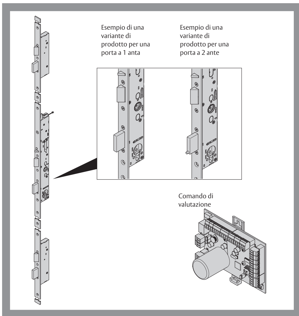
Fig. 1: Sistema di bloccaggio multiplo antipanico mFlipLock access/e-access
