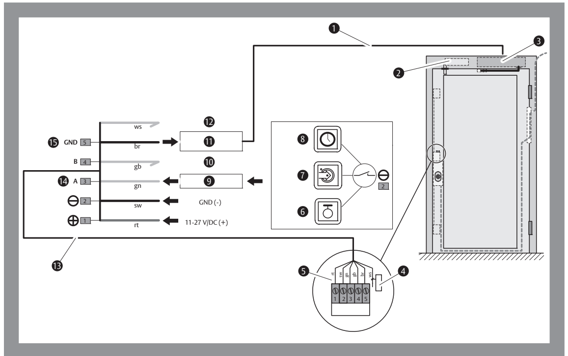
Abb. 10: Anschlussschema mFlipLock 25544PE-SV drive
