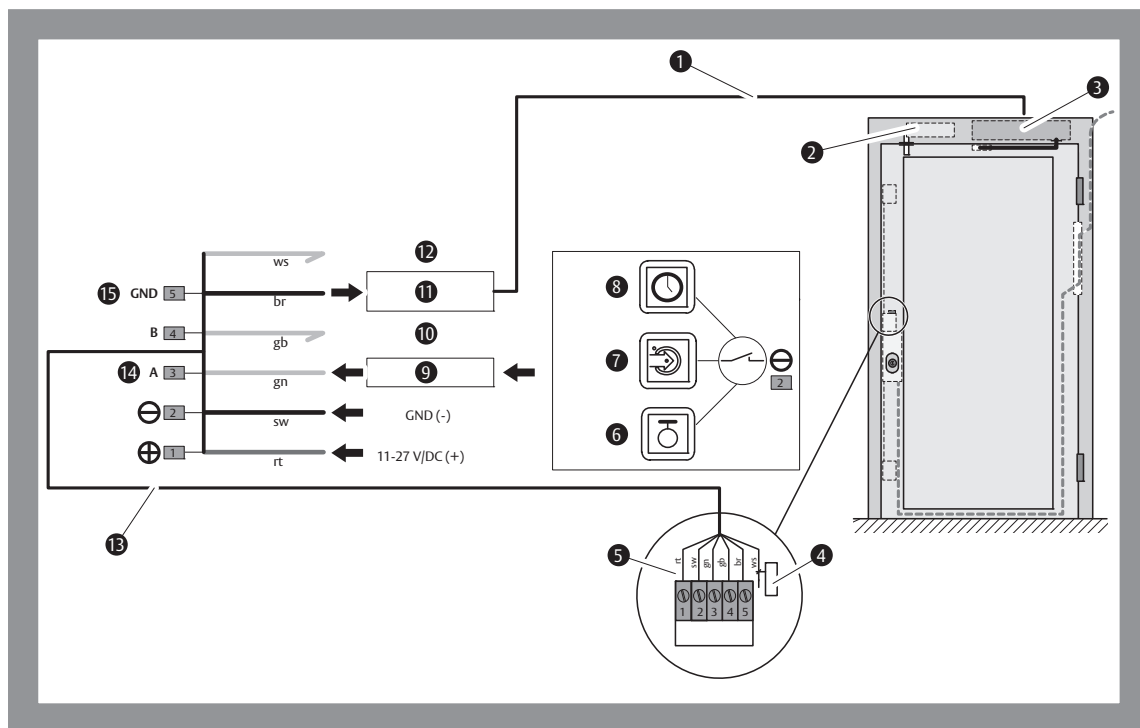
Abb. 11: Anschlussschema mFlipLock 26546PB-SV e-drive
