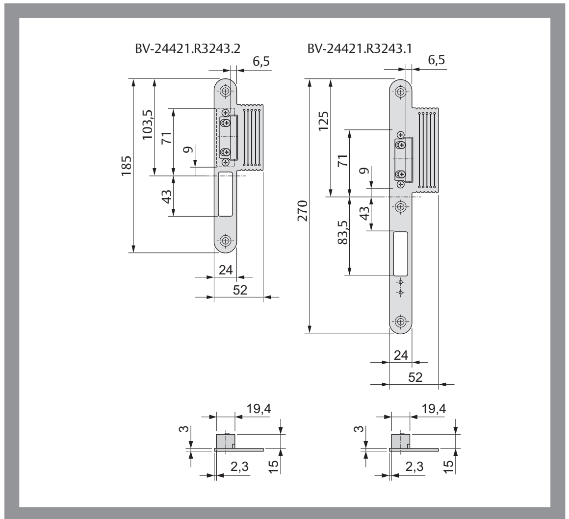
Abb. 11: Schließbleche für Holz
