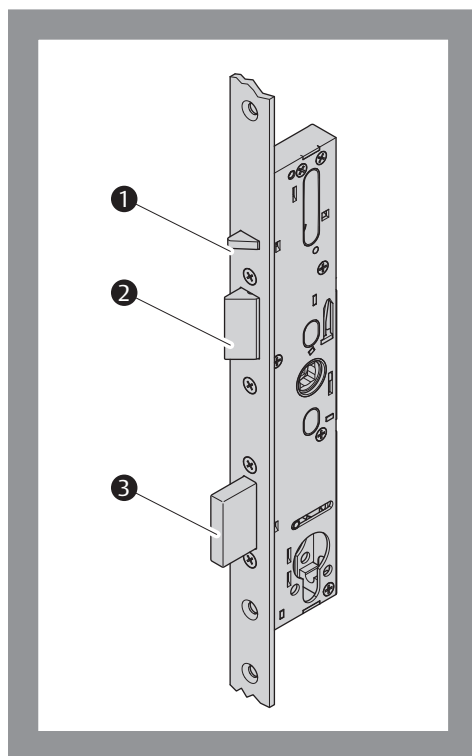
Fig. 5 : ① Pêne pilote ② Pêne demi-tour ③ Pêne dormant
