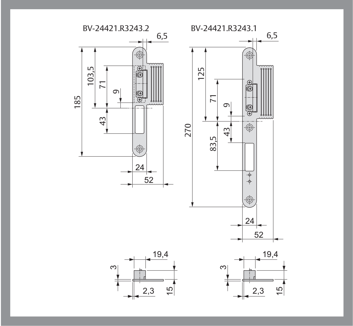
Fig. 11 : Têtières pour bois
