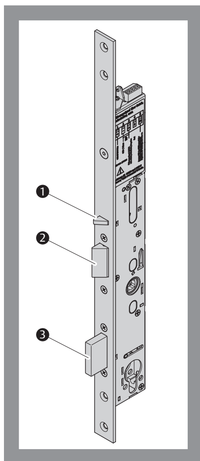
Fig. 5 : ① Pêne pilote ② Pêne demi-tour ③ Pêne dormant
