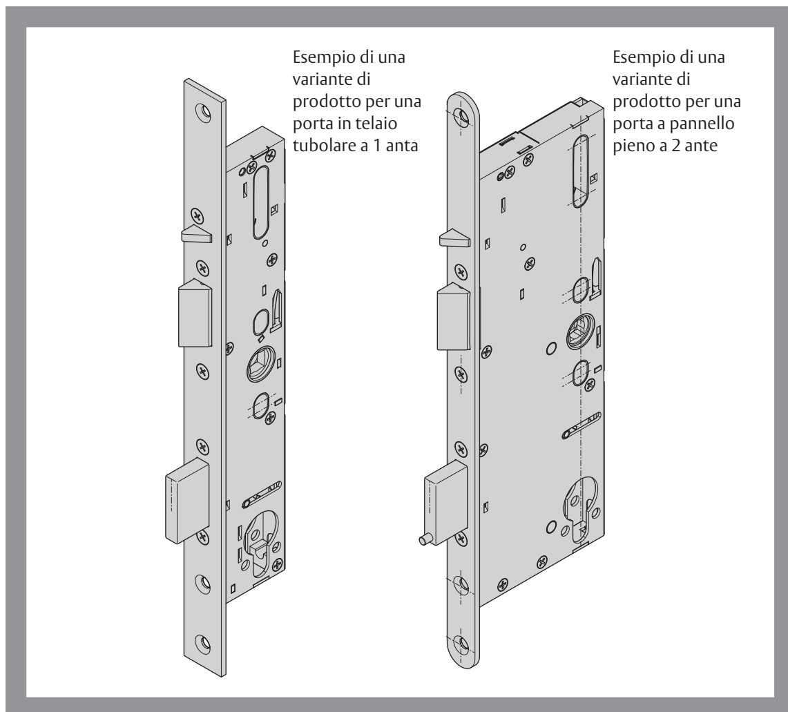
Fig. 1: Serratura a inserimento antipanico sFlipLock standard
