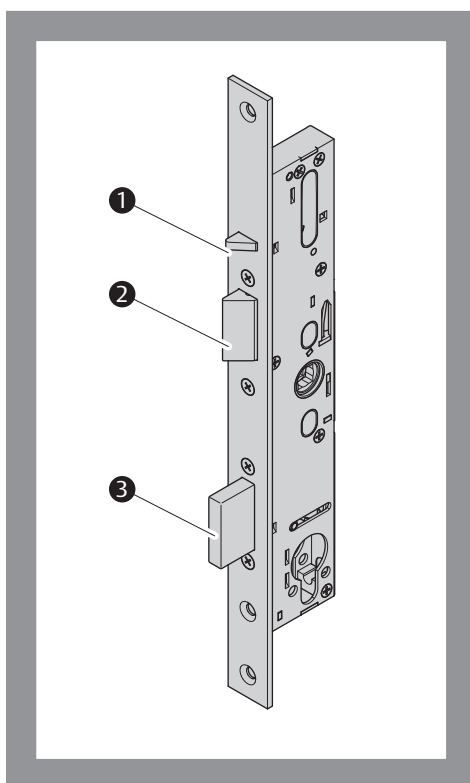
Fig. 5 : ① Pêne pilote ② Pêne demi-tour ③ Pêne dormant
