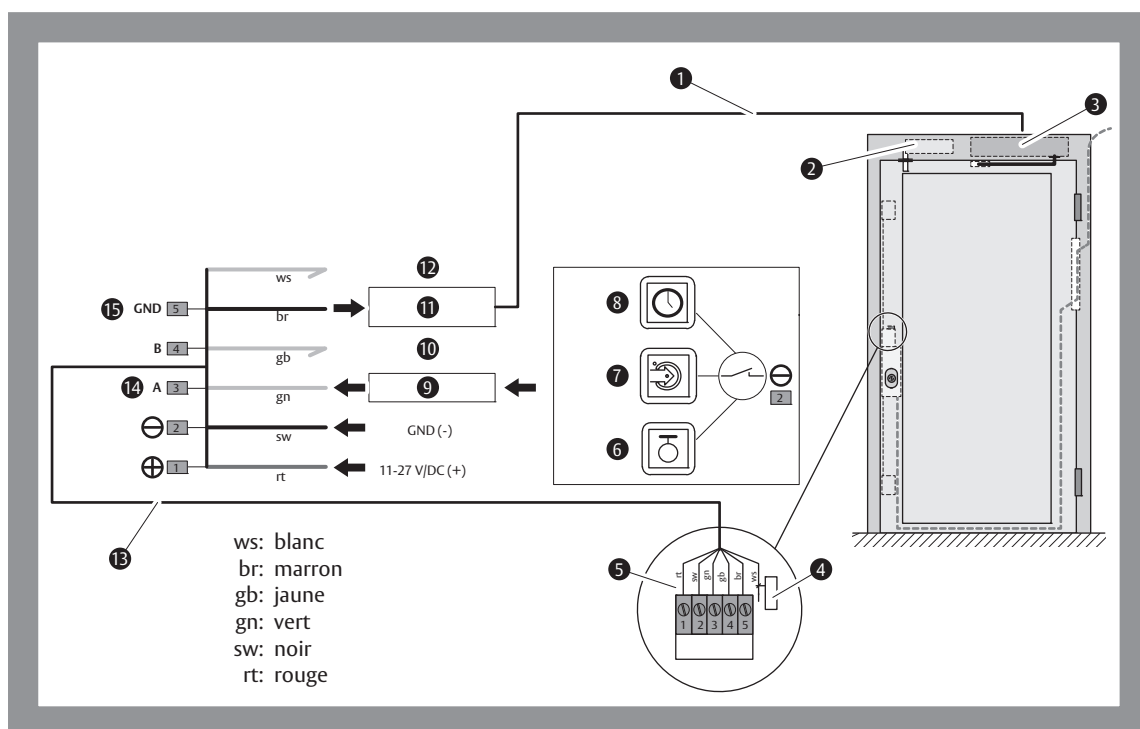
Fig. 11 : Schéma de raccordement sFlipLock 16546PB-SV drive
