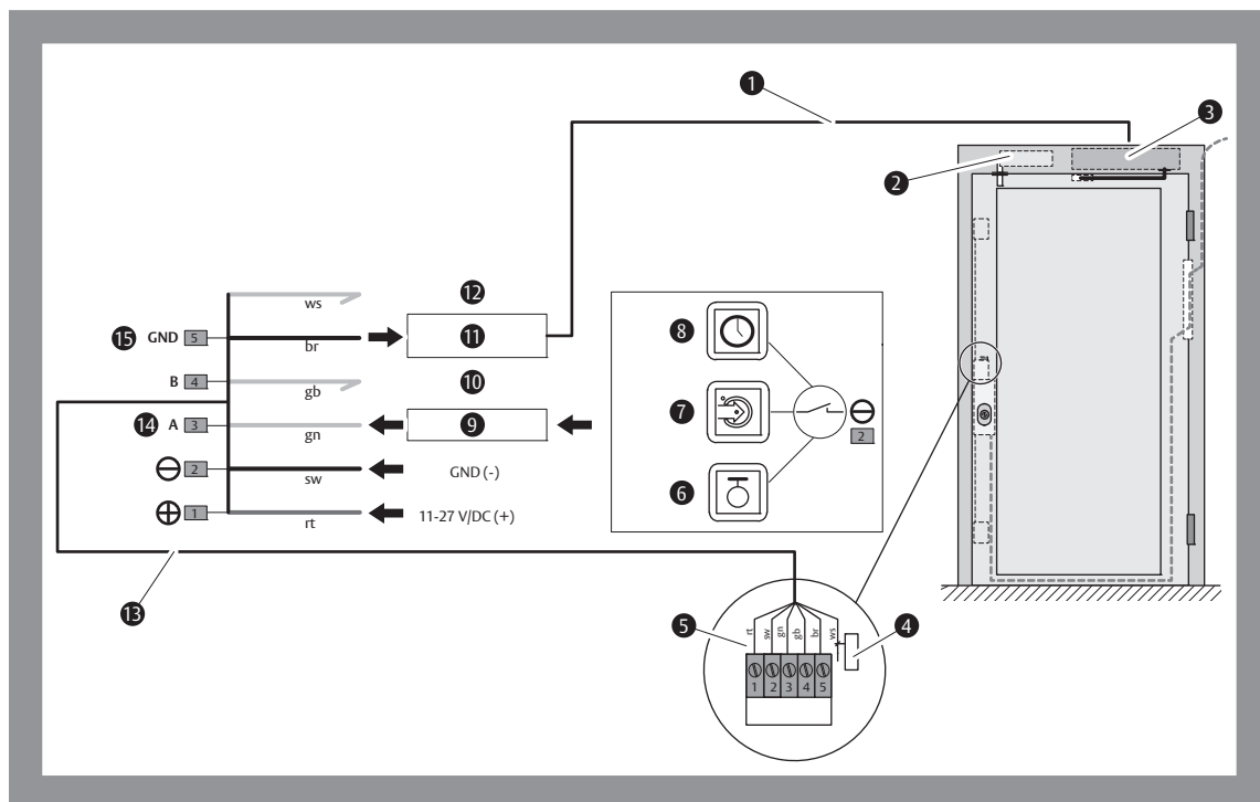
Abb. 10: Anschlusschema sFlipLock 15544PE-SV drive
