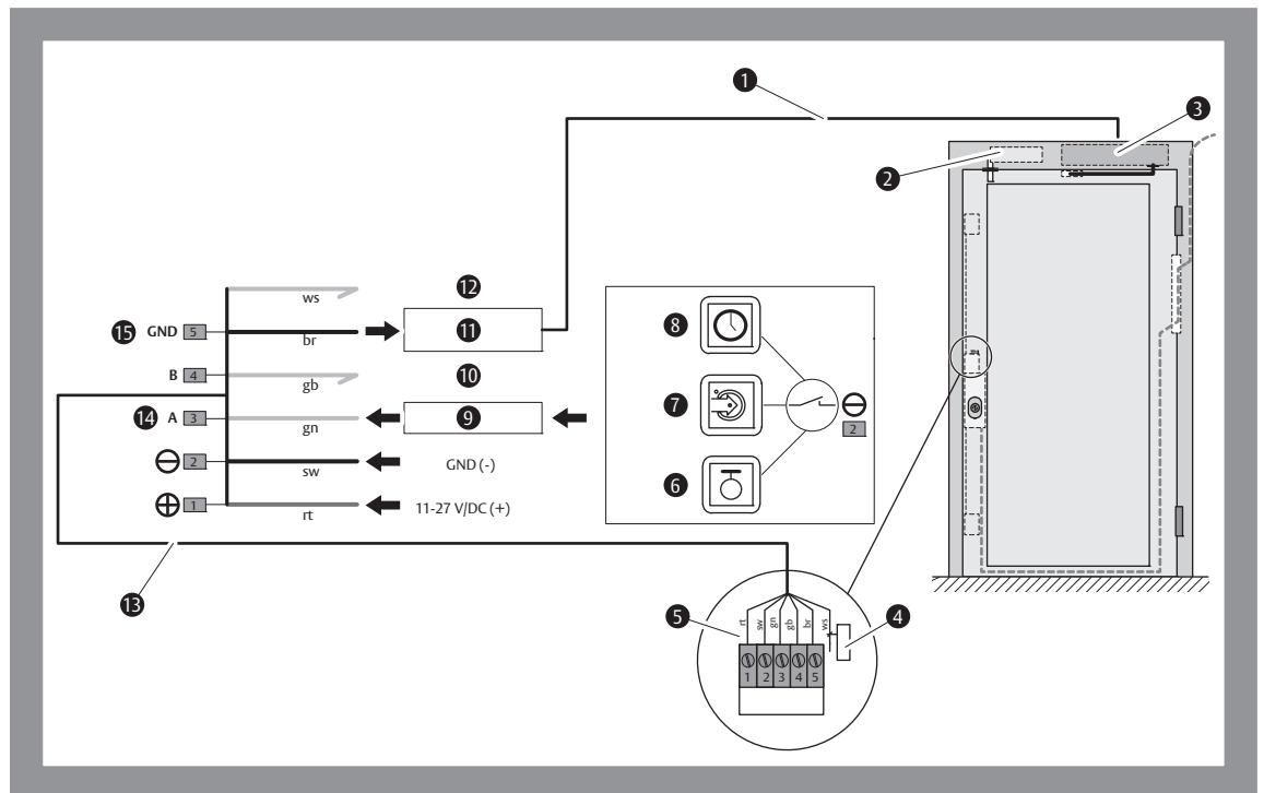
Abb. 11: Anschlussschema sFlipLock 16546PB-SV drive
