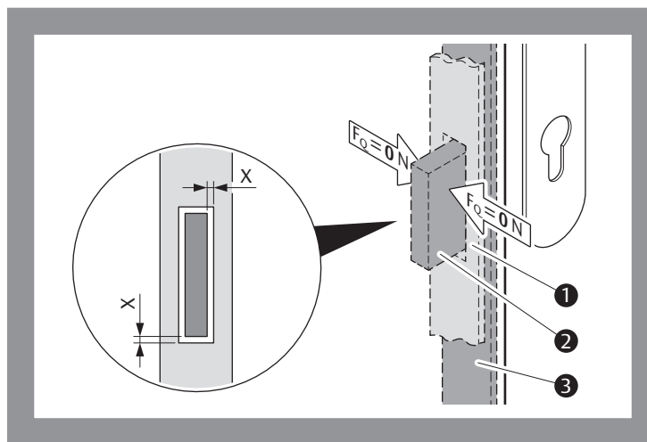
Abb. 8: Riegel ist frei von Querbelastungen ( F_Q )
