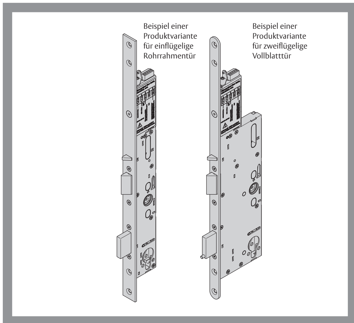
Abb. 1: Panik-Sicherheits- Einsteckschlösser sFlipLock drive/e-drive
