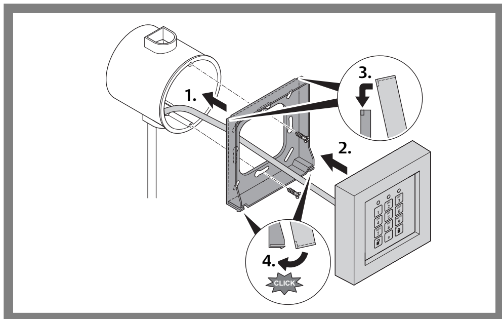
Abb. 2: Montage des SCALA Lesers
