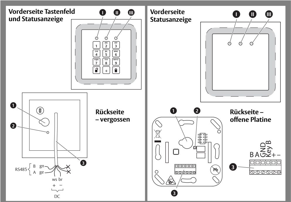
Abb. 1: SCALA Lesers – mit Tastenfeld und LED-Statusanzeige, die Platine ist vergossen, Anschluss über Kabel – mit LED Statusanzeige, die Platine ist offen, Anschluss über Schraubklemmleiste
