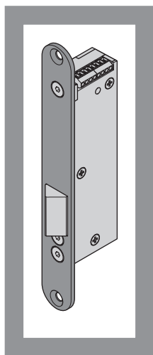
Abb. 1: Fluchttürverriegelung 352M
