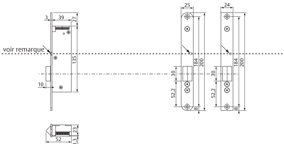
Têtières au niveau du verrouillage
