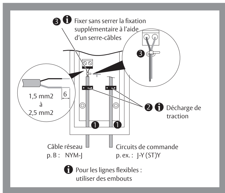
Fig. 2: Travaux préparatoires
