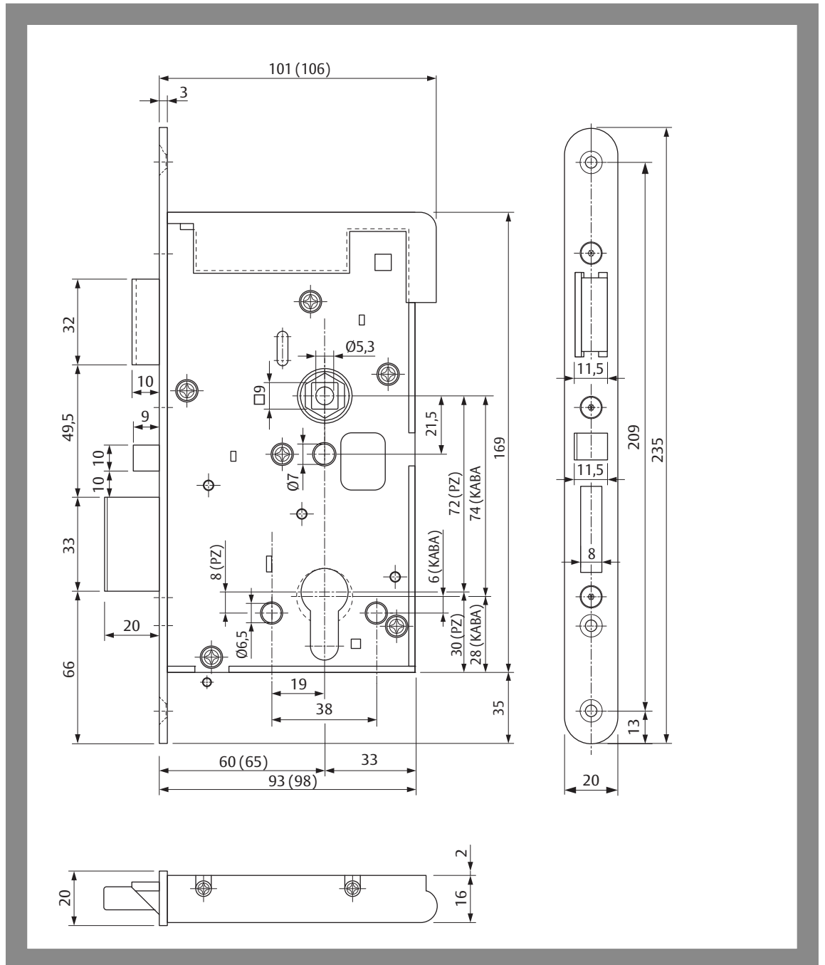
Abb. 10: Abmessungen des Sicherheitsschlosses 309 Vollblatt
