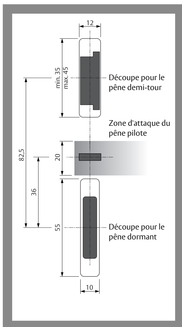
Fig. 9 : Dimensions pour la fabrication de têtes (côté dormant) sur site
