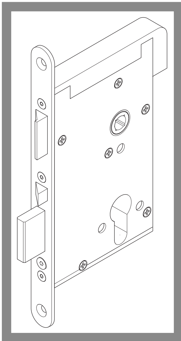
Abb. 1: Sicherheitsschloss 309
