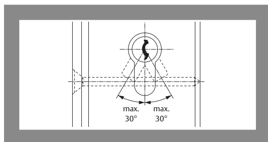
Fig. 8 : Position de retrait de la clé
