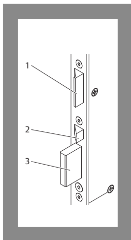
Fig. 5 : 1 Pêne demi-tour 2 Pêne pilote 3 Pêne dormant
