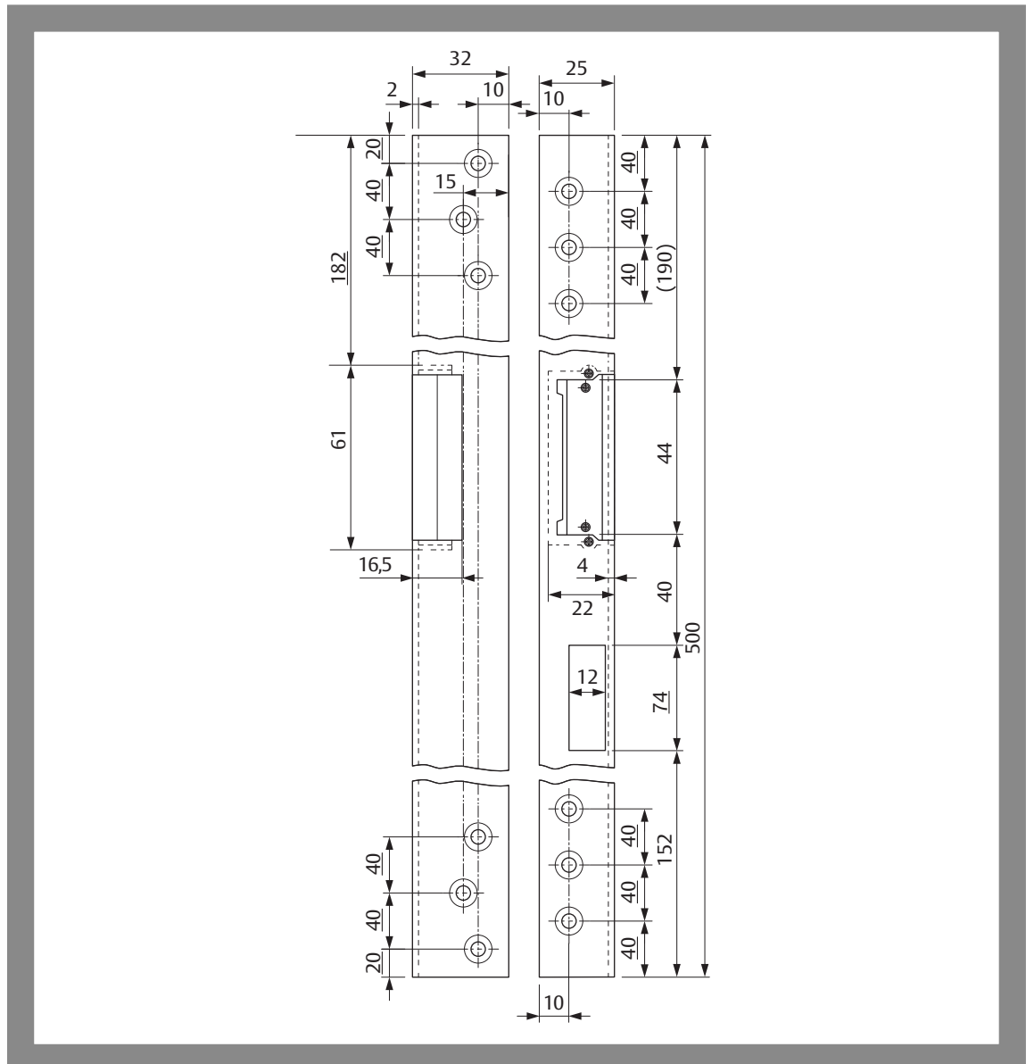
Fig. 13 : Tête d'angle de sécurité
