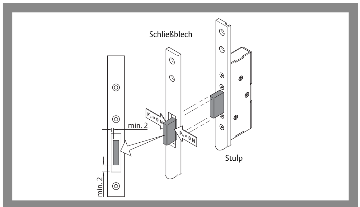
Abb. 6: Riegel nach Montage frei von Querbelastungen
