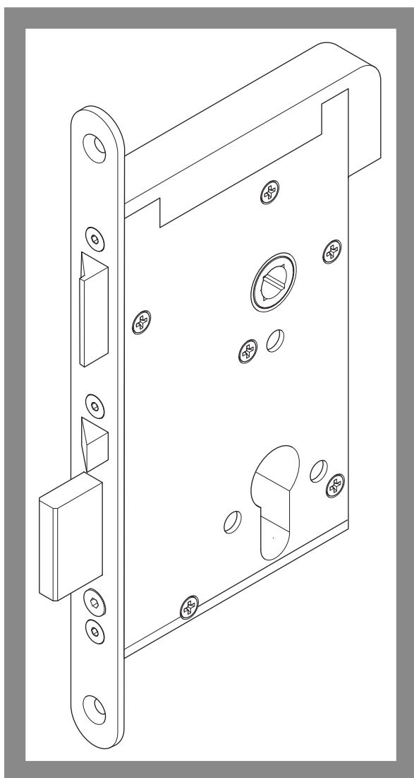
Fig. 1: Serrure de sécurité 309
