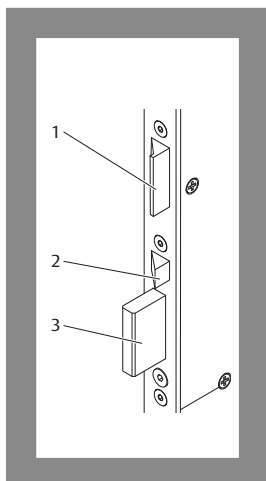
Abb. 5: 1 Schlossfalle 2 Steuerfalle 3 Riegel
