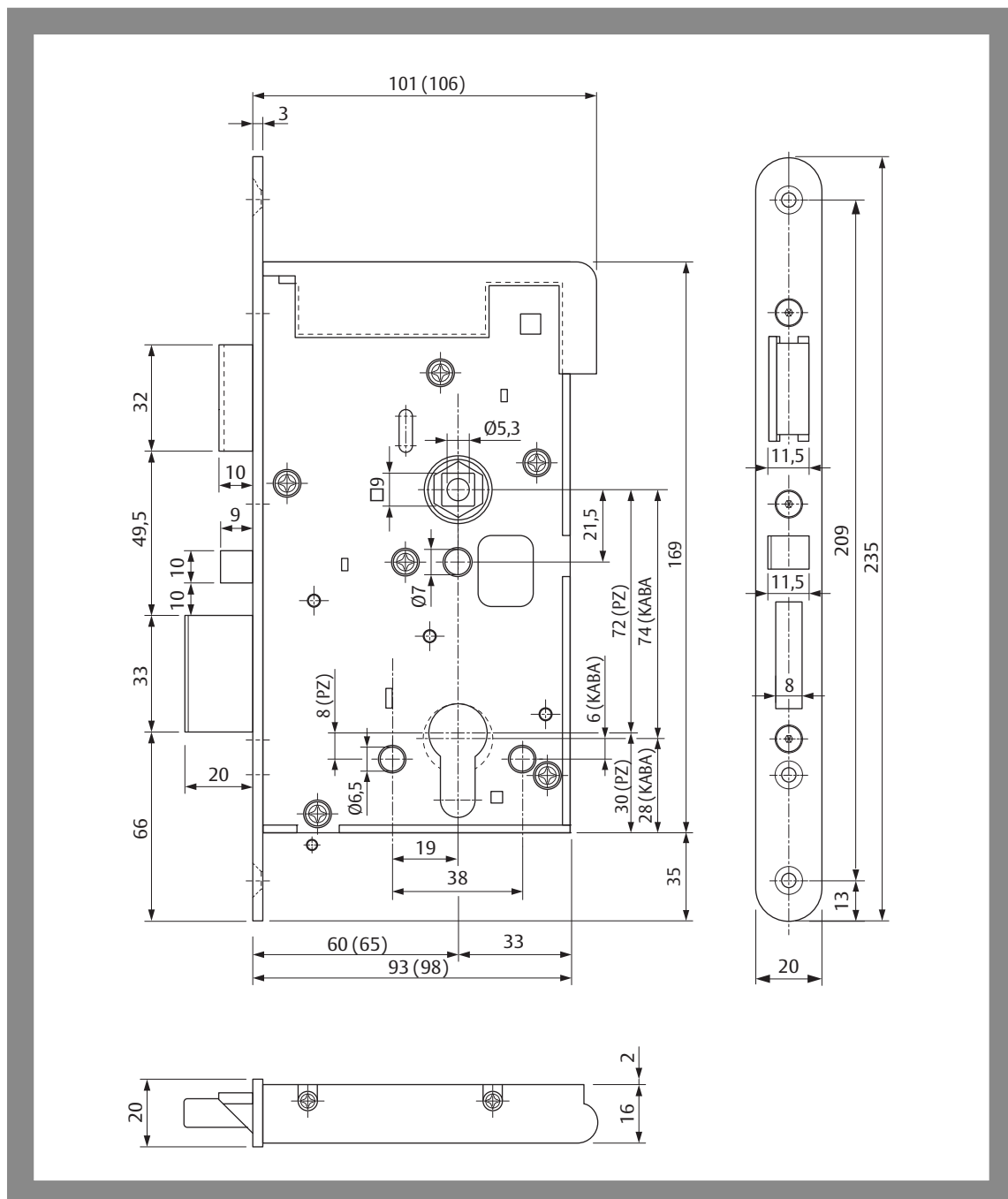
Fig. 10 : Dimensions de la serrure de sécurité 309 - portes pleines
