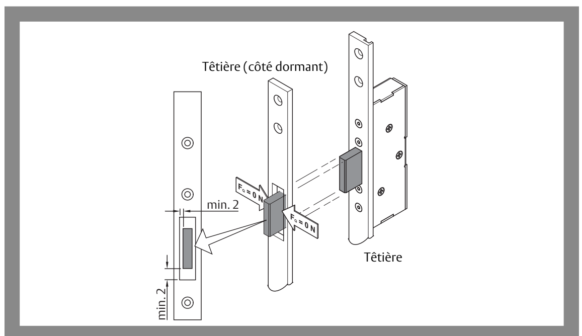
Fig. 6 : Absence de contraintes transversales sur le pêne dormant après le montage
