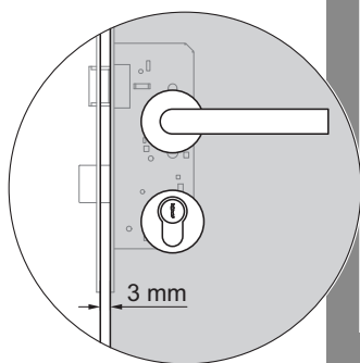
Fig. 4: Jeu de feuillure
