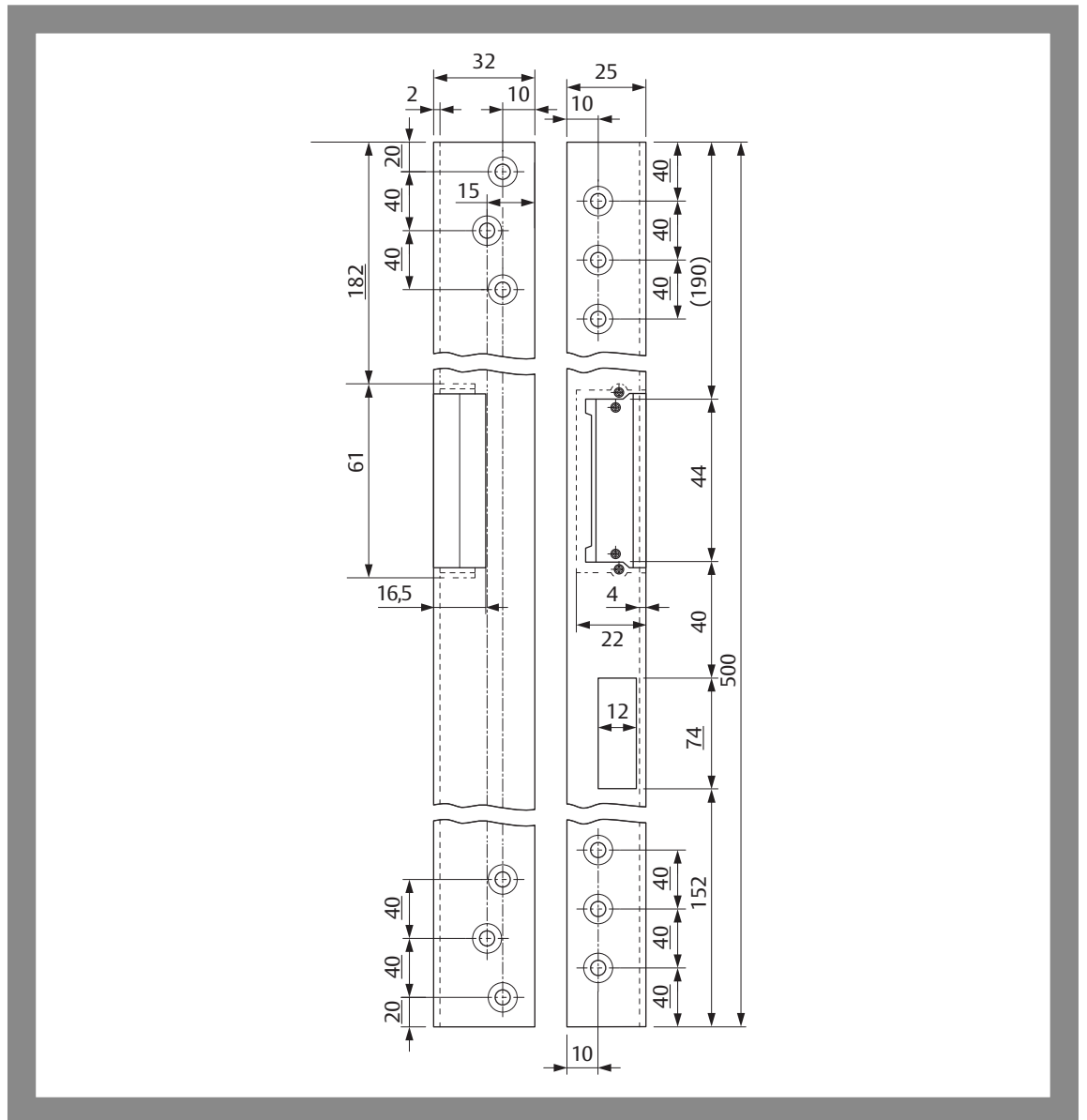
Abb. 13: Sicherheitswinkelschließ- blech
