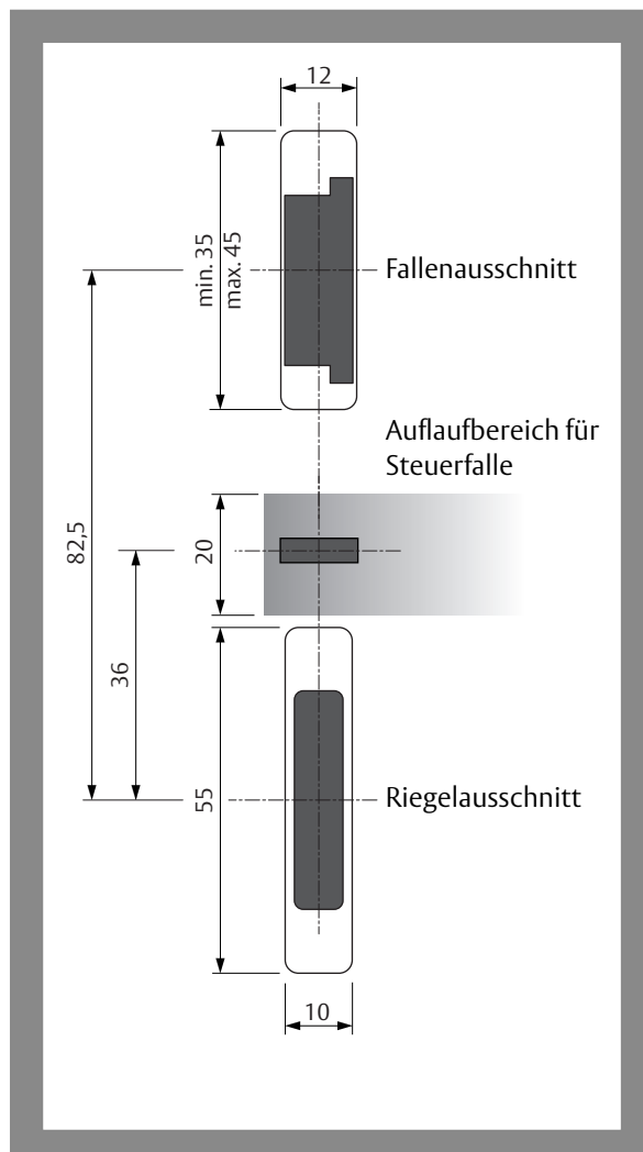
Abb. 9: Bemaßung für die Fertigung bauseitiger Schließbleche
