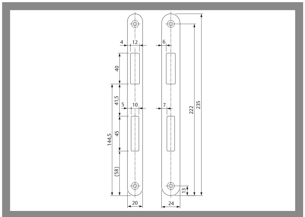
Abb. 11: Flachschließblech, verschiedene Breiten
