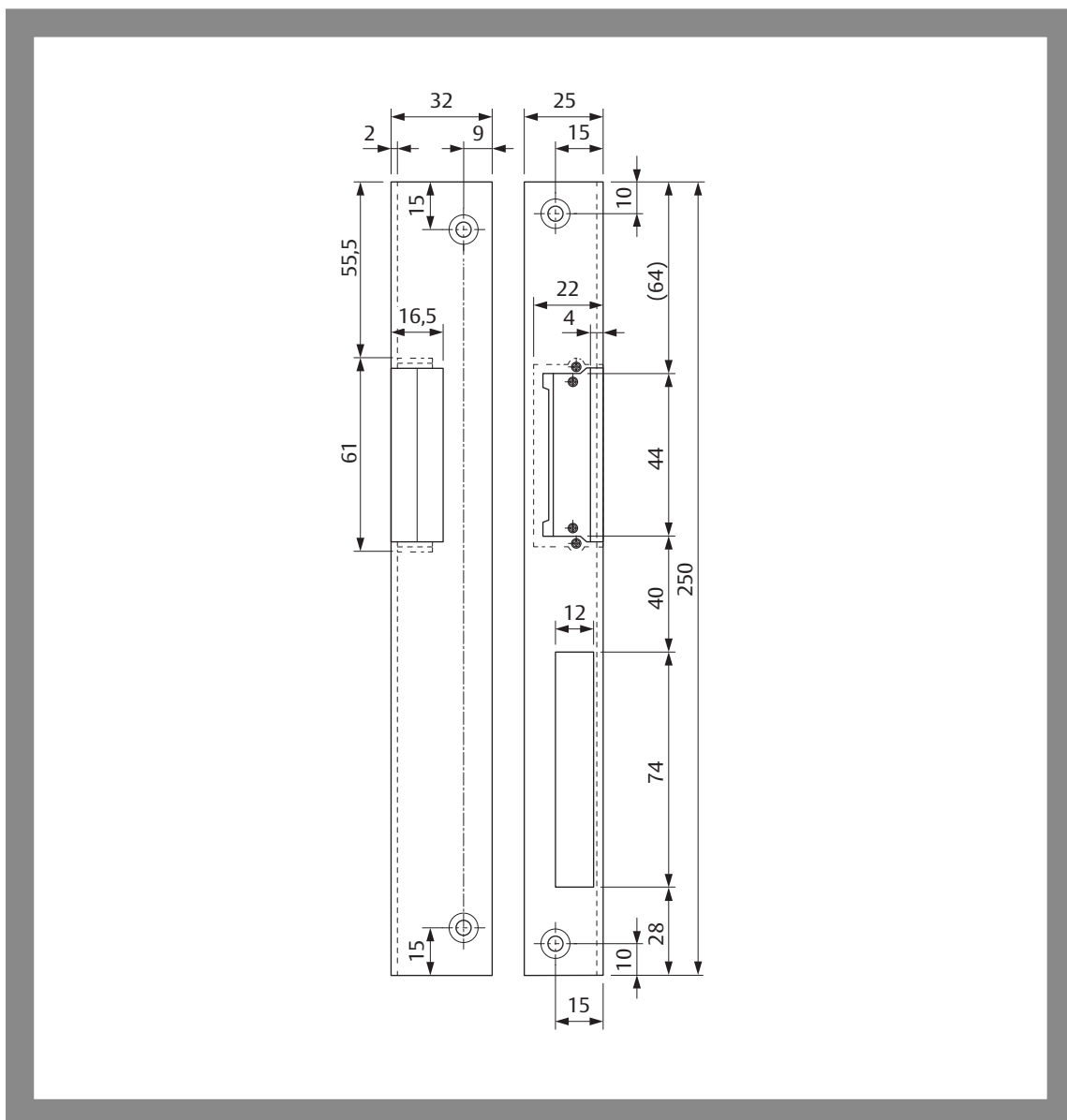
Fig. 12 : Têtière d'angle
