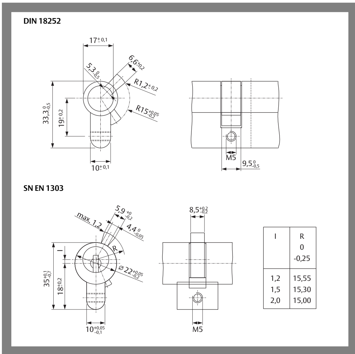
Fig. 18: Dimensioni della Cilindri di chiusura secondo la norma DIN 18252 o SN EN 1303SN
