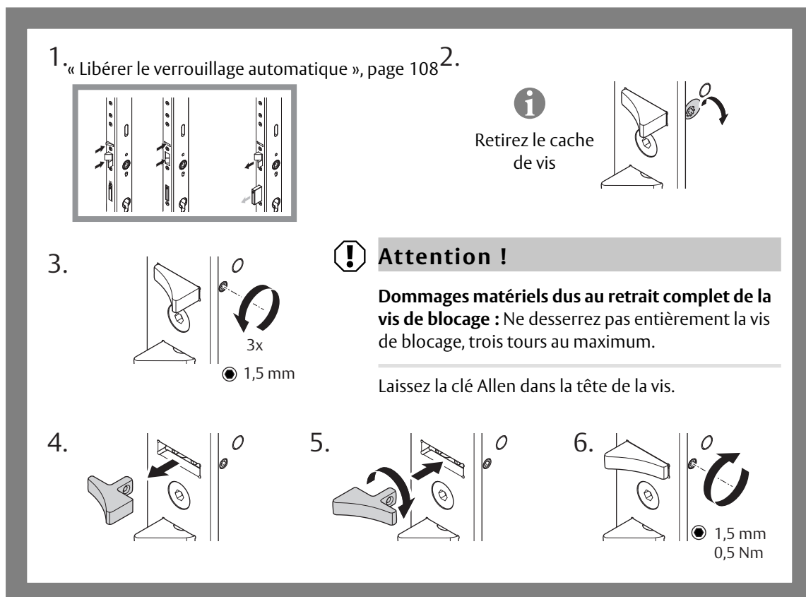
Fig. 9: Inversion de la position du pêne pilote
