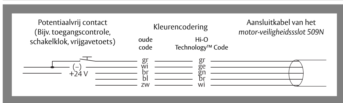
Afb. 14: Aansluitschema
