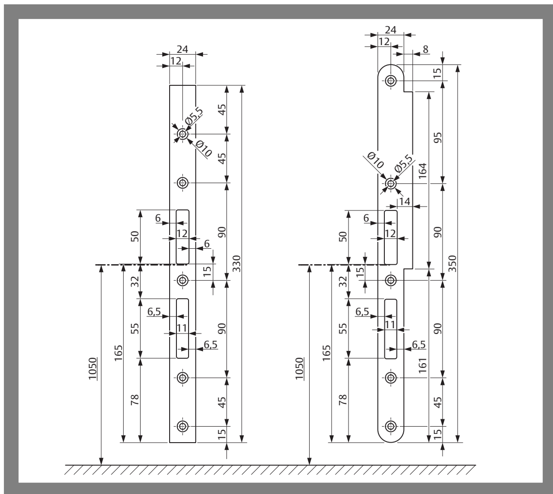
Fig. 19: Frontali
