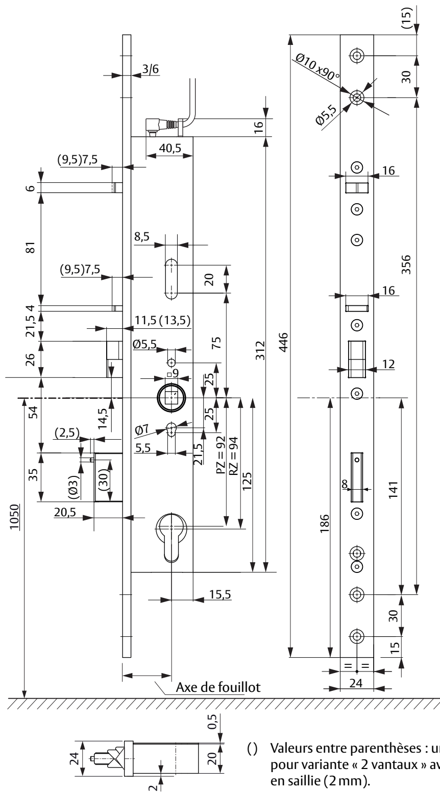
Fig. 17 : Dimensions de la serrure de sécurité motorisée 509N
