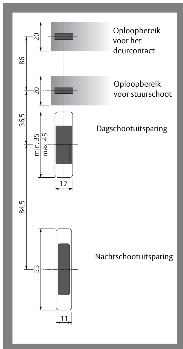
Afb. 16: Maatvoering voor het vervaardigen van lokale sluitplaten
