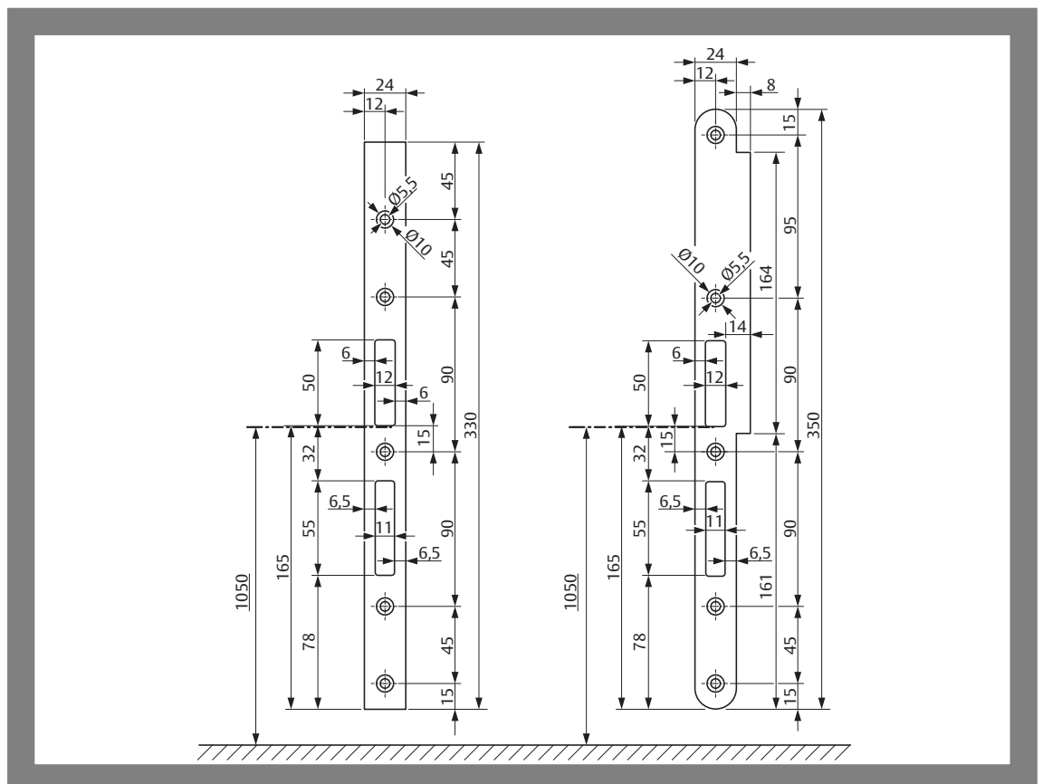
Abb. 19: Schließbleche
