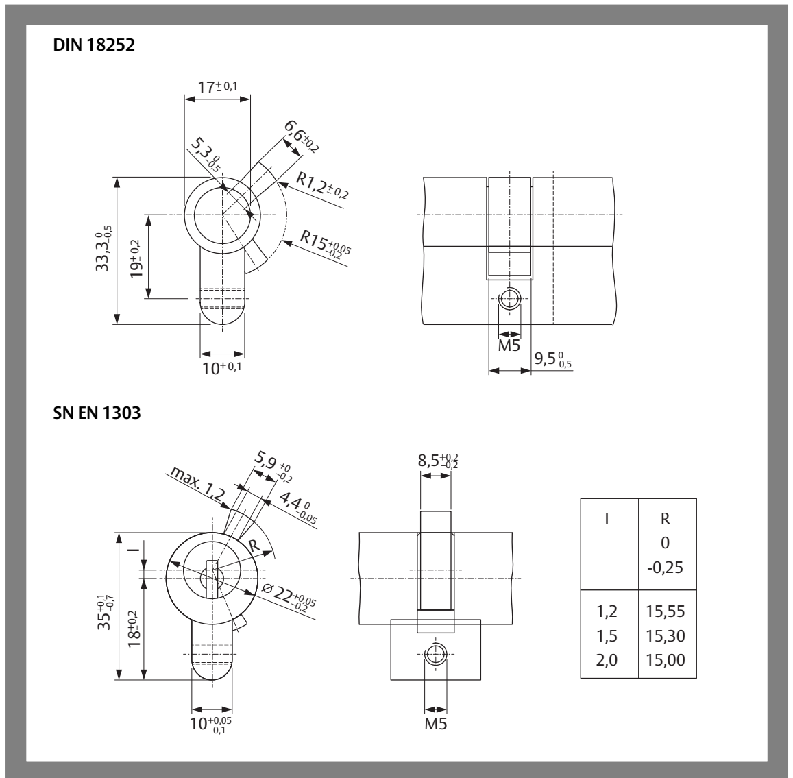
Abb. 18: Abmessungen der Schließzylinder nach 18252 und SN EN 1303
