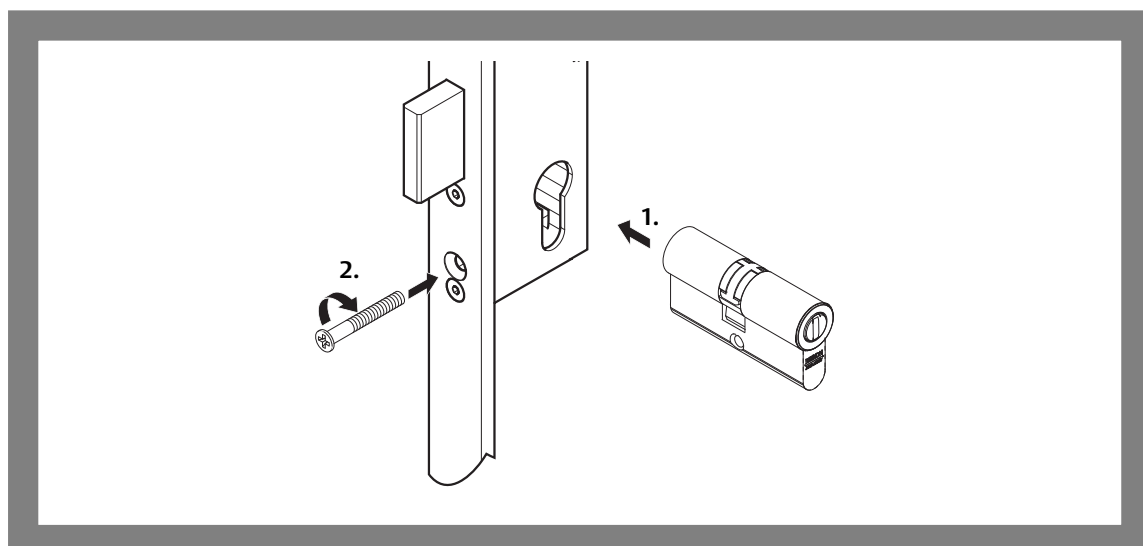
Afb. 13: Een profielcilinder monteren
