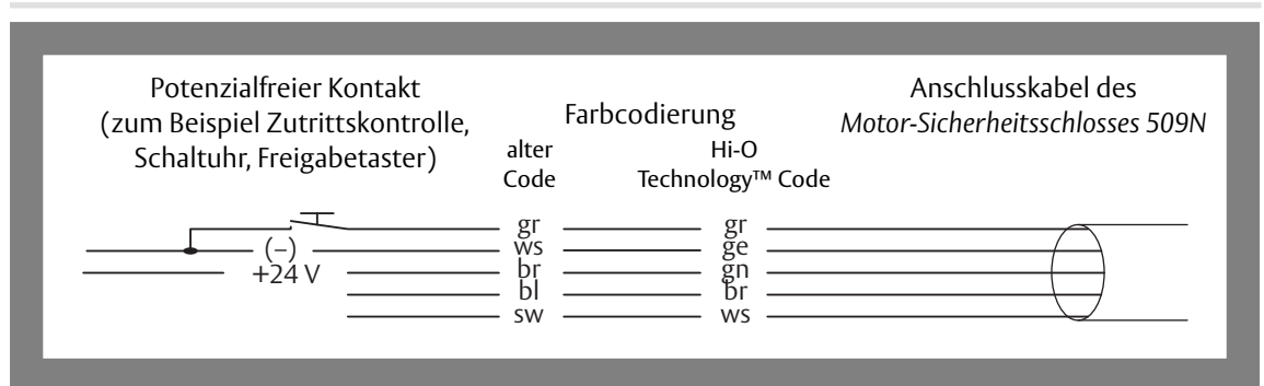
Abb. 14: Anschlussplan
