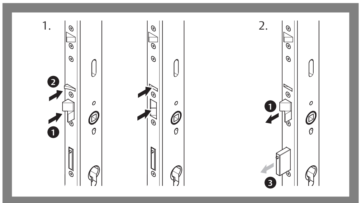
Abb. 7: Selbstverriegelung auslösen
