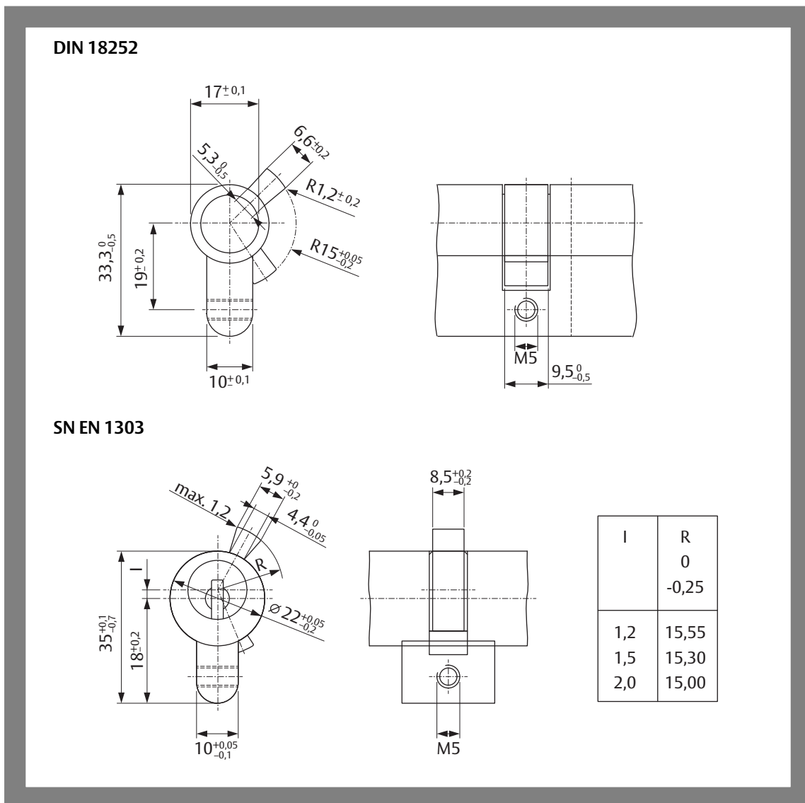
Fig. 18: Dimensions de Cylindre de fermeture selon la norme DIN 18252 ou SN EN 1303
