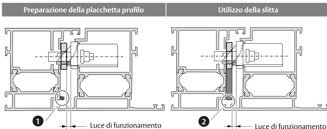
Fig. 15: Rilavorazione della placchetta profilo e utilizzo della slitta
