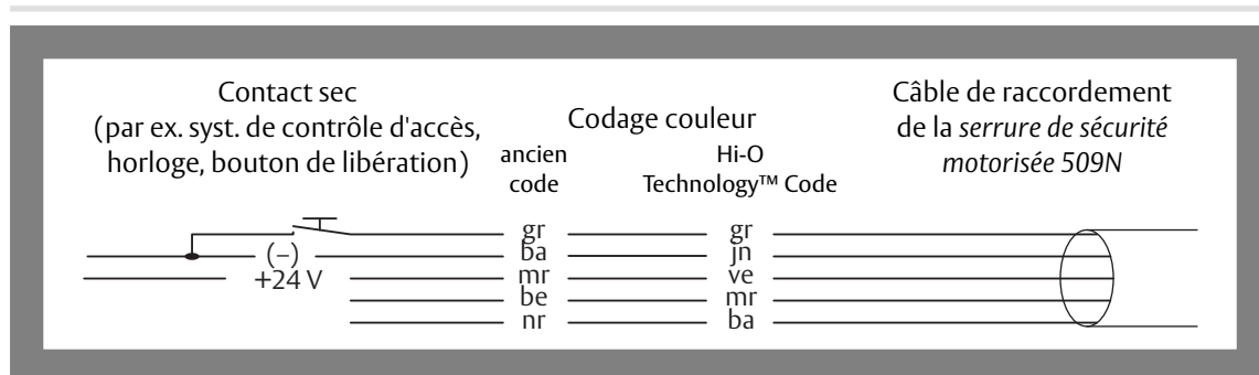
Fig. 14 : Plan de connexion
