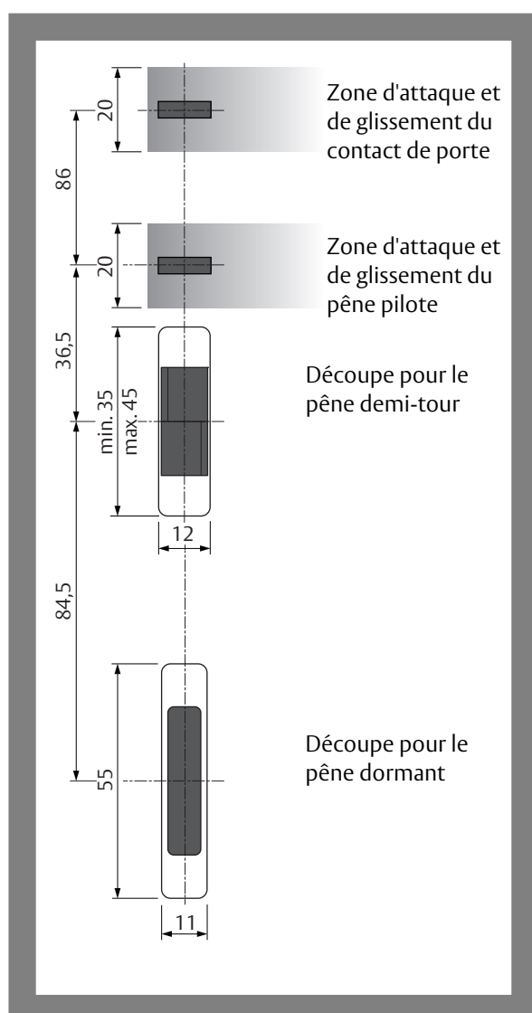
Fig. 16 : Dimensions pour la fabrication de têtes (côté dormant) sur site
