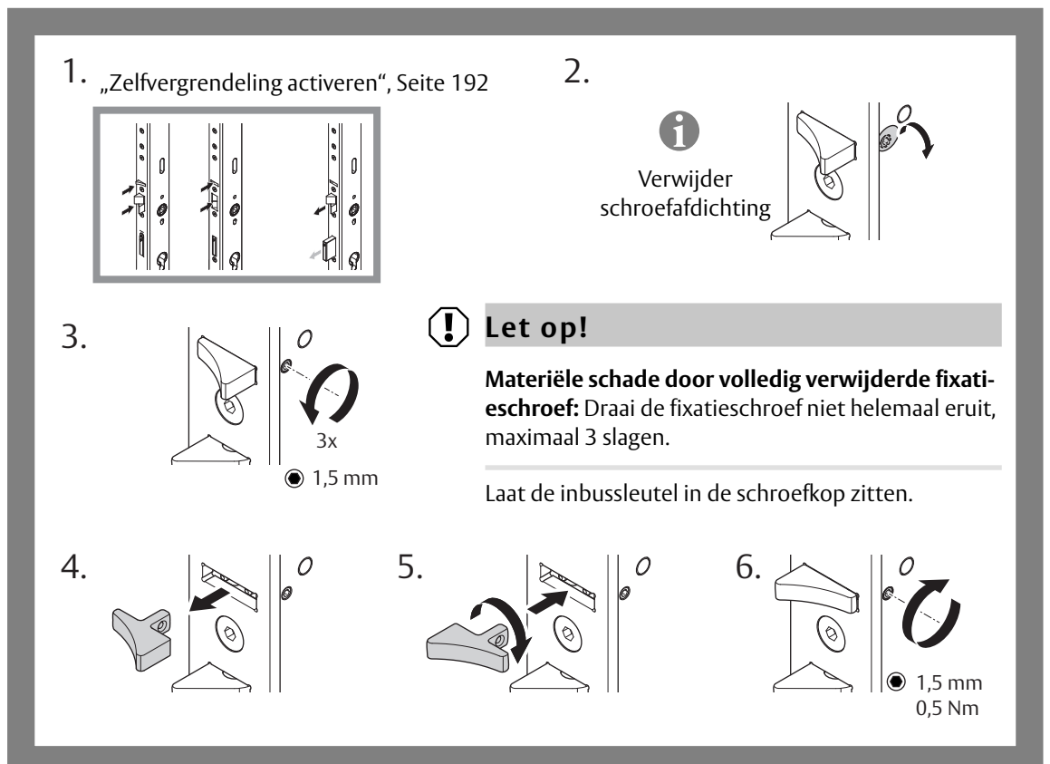
Afb. 9: Stuurschoot omdraaien
