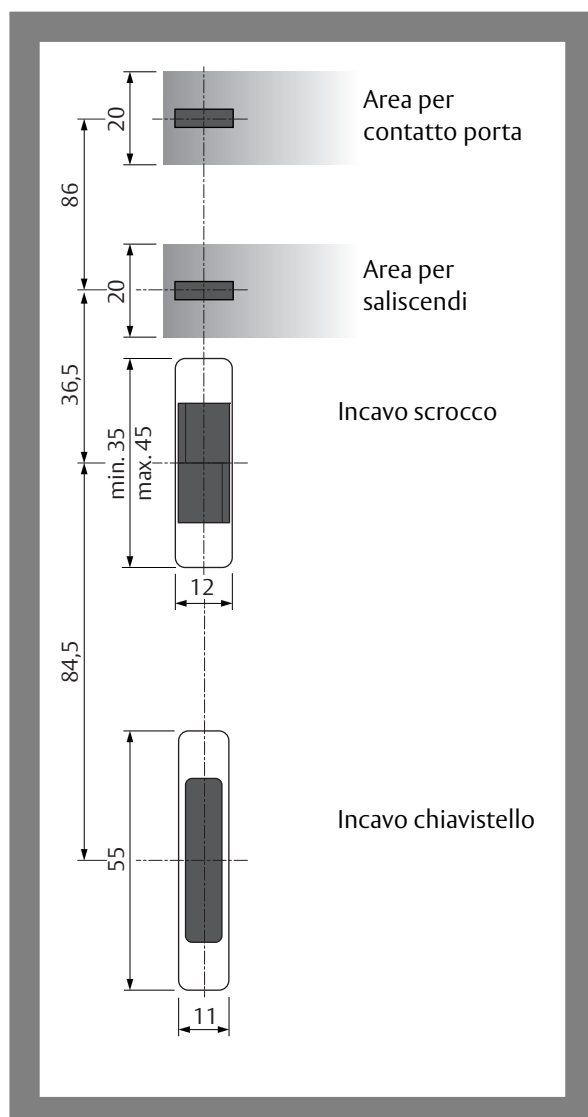
Fig. 16: Dimensionamento per la lavorazione dei frontali in loco
