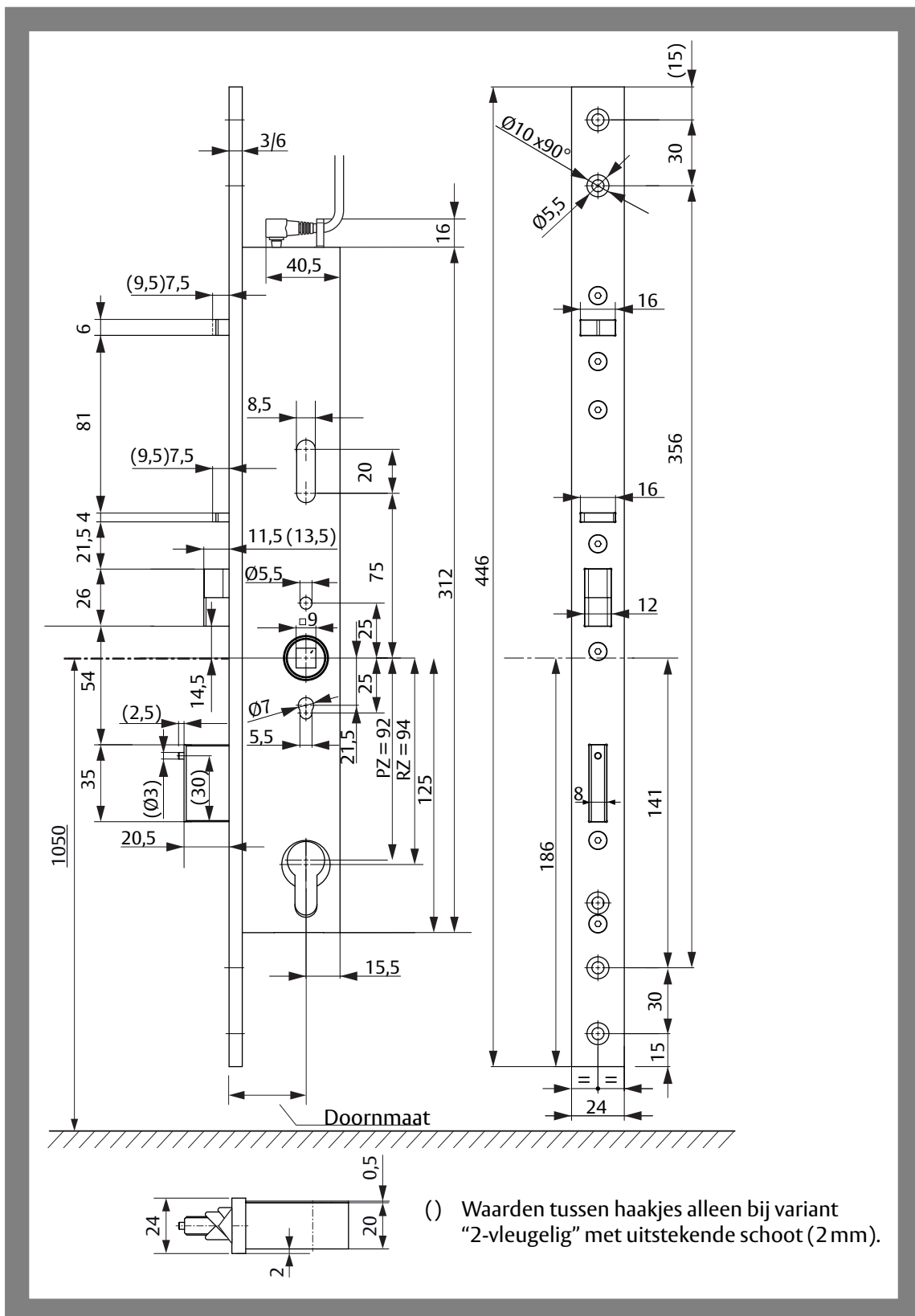
Afb. 17: Afmetingen van het motor-veiligheidsslot 509N
