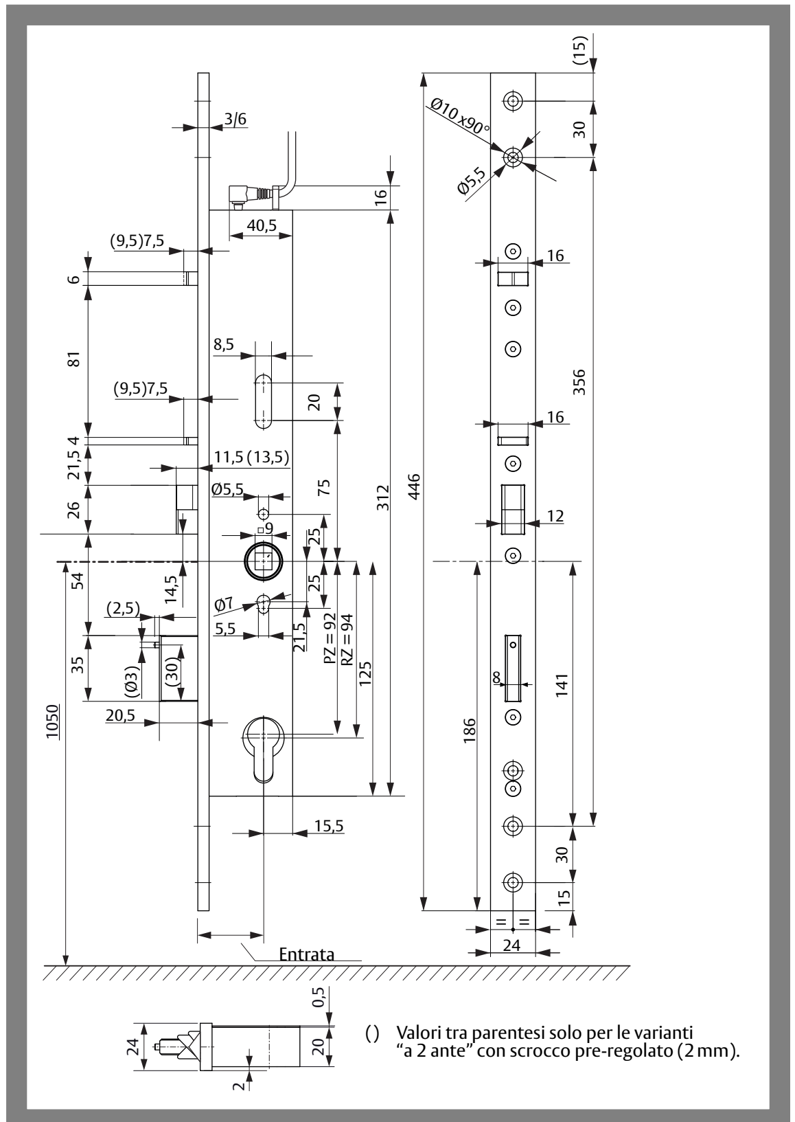
Fig. 17: Dimensioni della serratura motorizzata 509N
