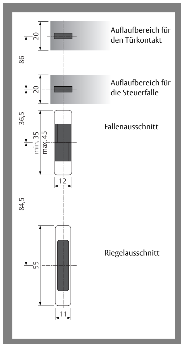
Abb. 16: Bemaßung für die Fertigung bauseitiger Schließbleche
