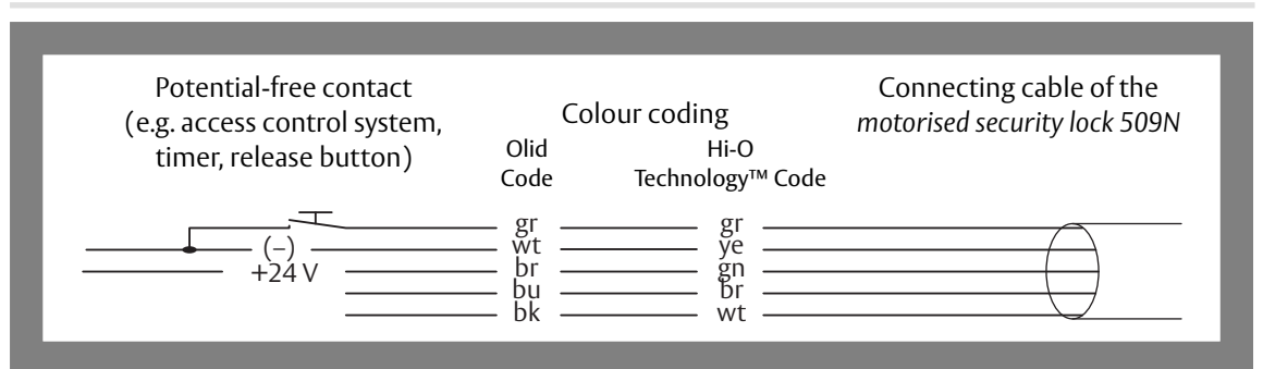
Fig. 14: Wiring diagram
