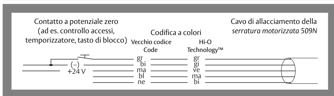
Fig. 14: Schema di collegamento
