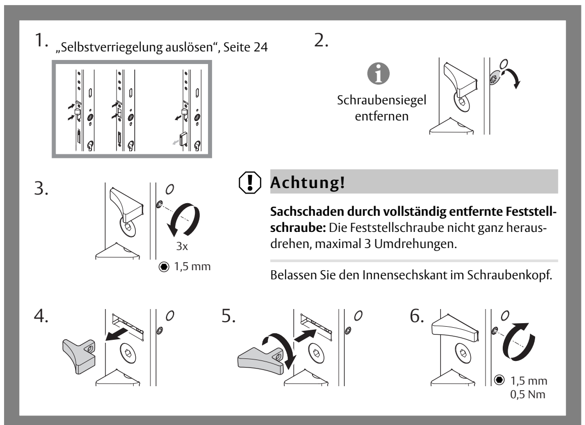
Abb. 9: Steuerfalle drehen
