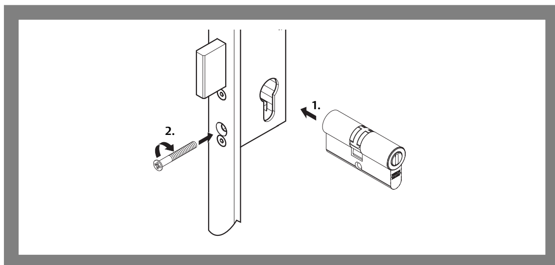
Fig. 13: Montaggio di un cilindro profilato
