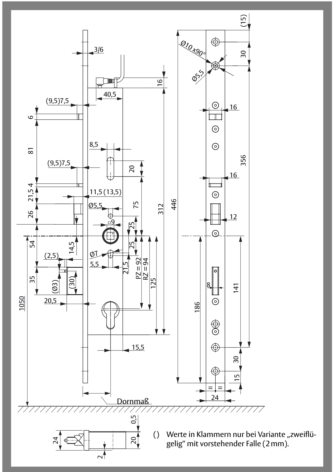
Abb. 17: Abmessungen des Motor- Sicherheitsschlosses 509N
