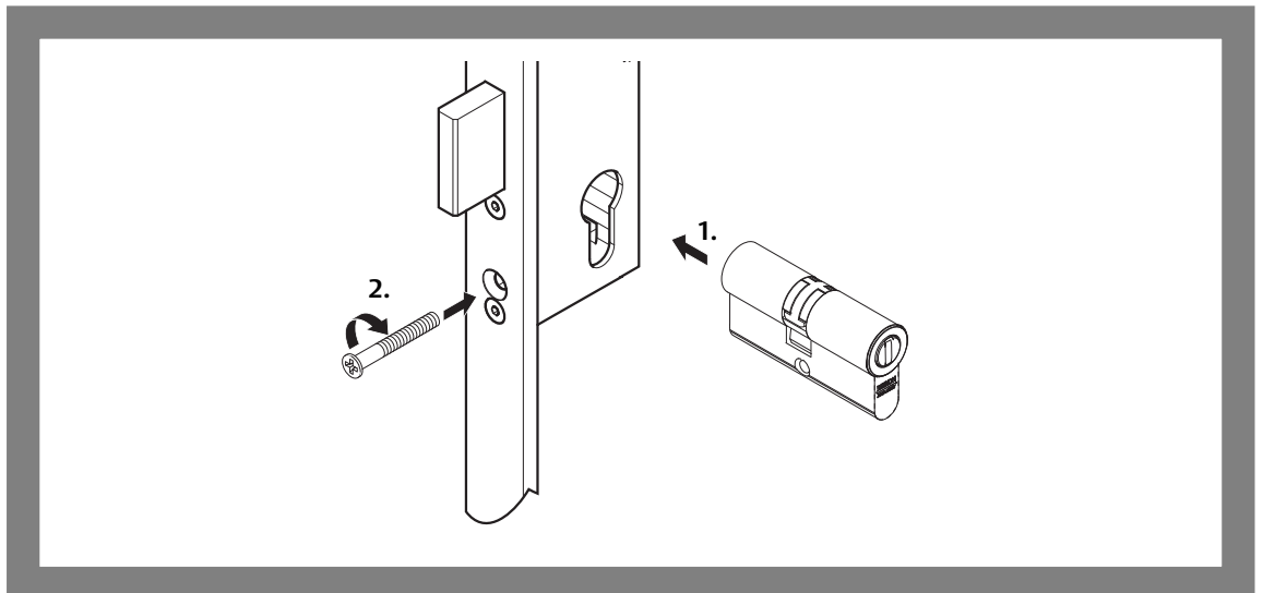
Abb. 13: Einen Profilzylinder montieren
