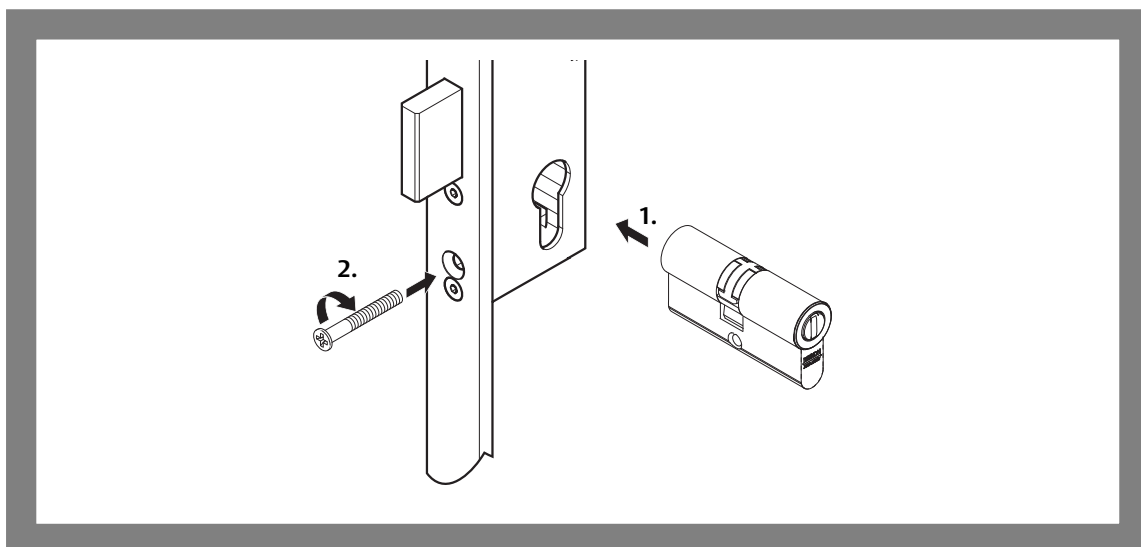
Fig. 13 : Monter un cylindre profilé
