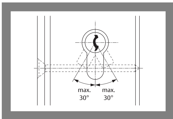
Fig. 12: Position de retrait de la clé
