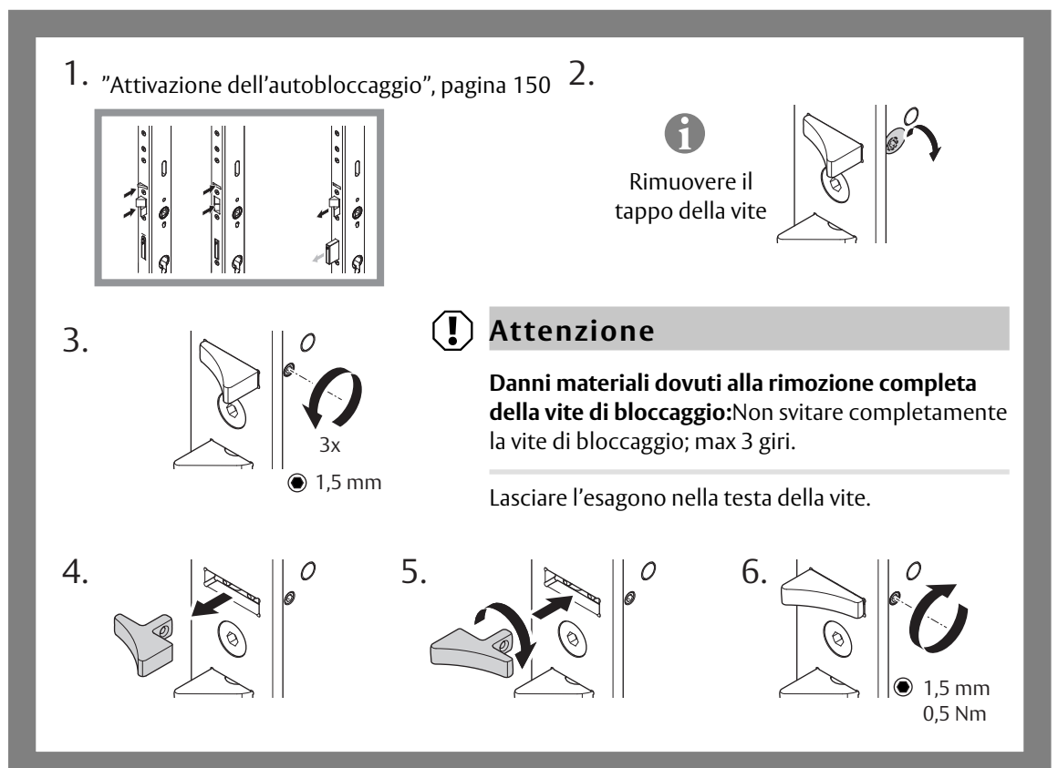
Fig. 9: Inversione dello scrocco di comando
