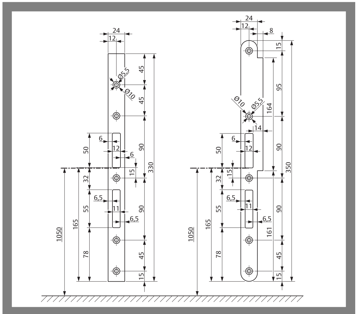
Fig. 19: Têtières
