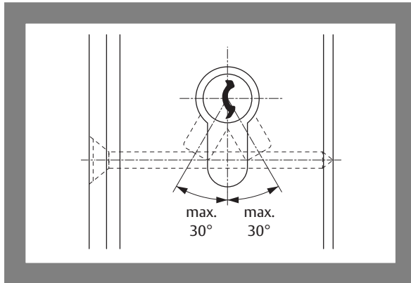
Abb. 12: Schlüsselabzugsstellung
