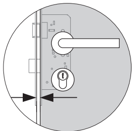
Fig. 3: Rebate gap
