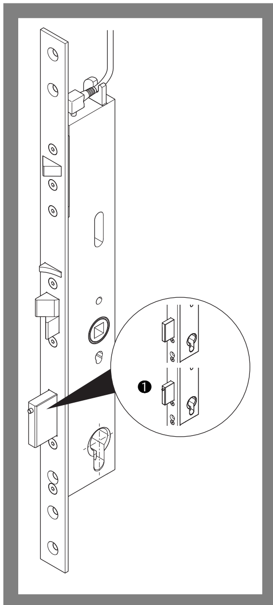
Afb. 1: Motor-veiligheidslot 509N
