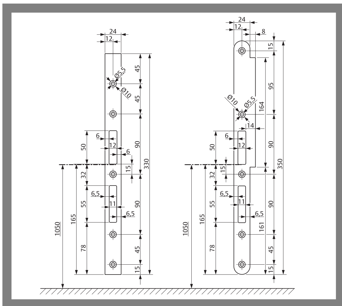
Afb. 19: Sluitplaten
