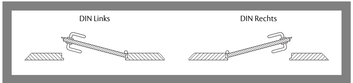
Abb. 8: Schlosstypen nach DIN Links und DIN Rechts
