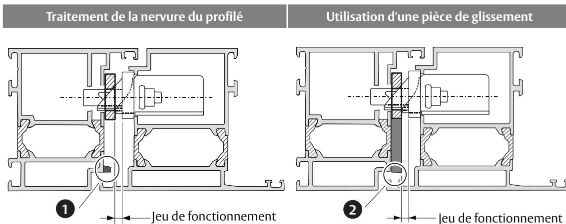
Fig. 15 : Post-traitement de la nervure de profilé et utilisation d'une pièce de glissement
