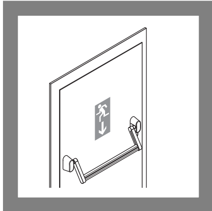
Abb. 10: Eine Panikfluchttür nach EN 1125
