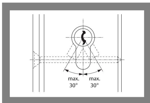
Fig. 12: Posizioni di estrazione chiave
